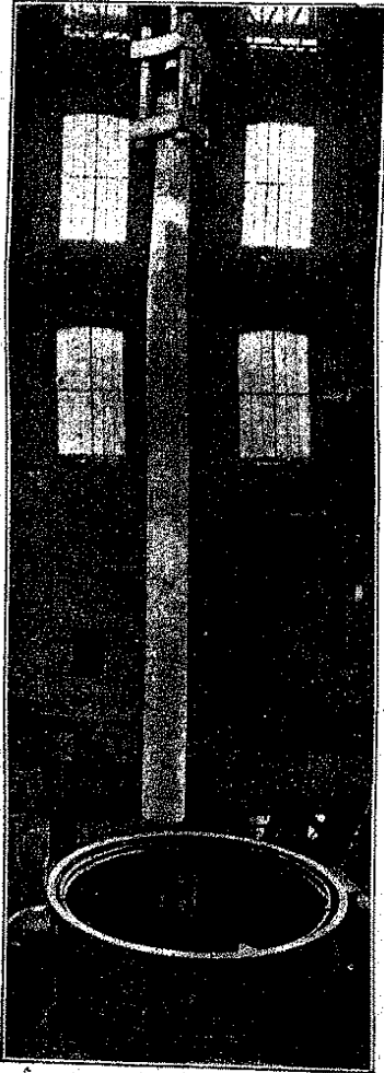
هذه صورة ازال ماسورة المدفع في بئر من الزيت البارد لتقسيتها وهي لا تزال في درجة الاحرار من الجو
